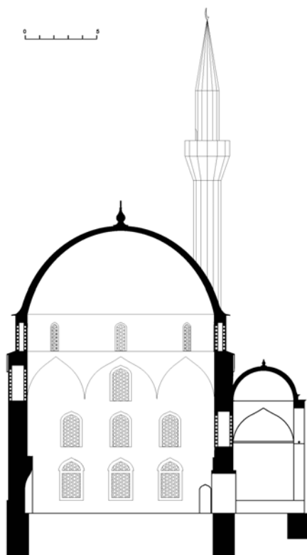
Hosszmetszet
