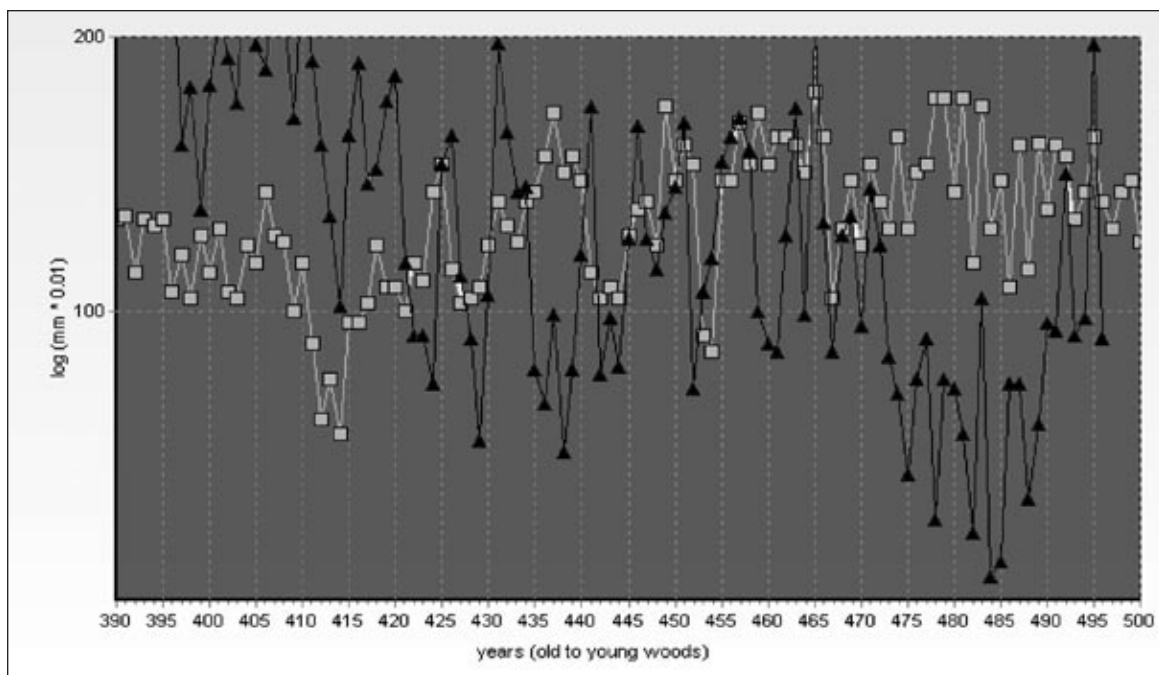
26. kép: A délnémet tölgykronológia (□) és a Tisza-mederből származó tölgyfácölöpből vett 6. minta (▲) évgűrűgörbéinek összehasonlítása.
