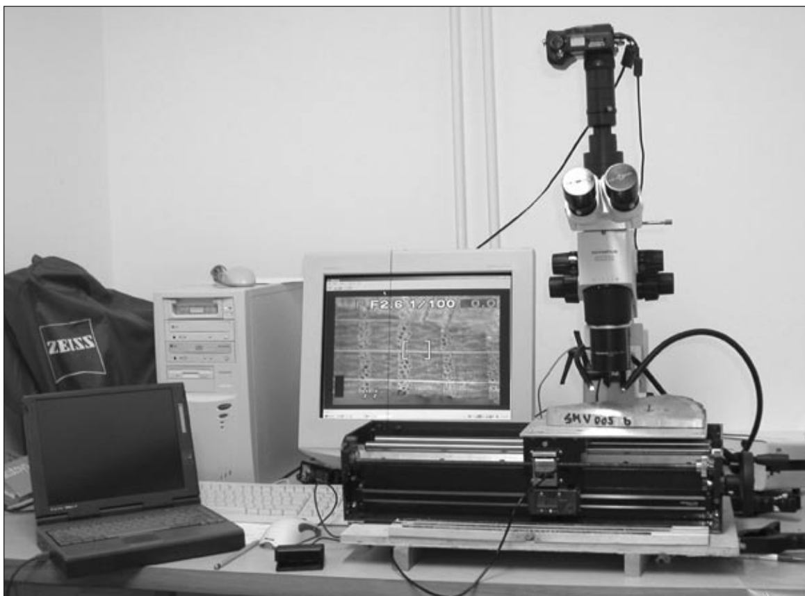
24. kép: Az évgyűrűszélességek mérésére szolgáló berendezés számítógéppel összekötve. Fig. 24: The instrument for measuring the annual-ring widths connected with a computer.
