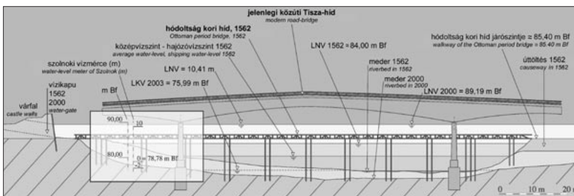
30. kép: A Tisza keresztmetsvénye a török kori és a mai medrekkel, hidakkal, valamint a fontosabb vízszintekkel (LNV = legnagyobb vízszint, LKV = legkisebb vízszint, Bf = Balti-tengerszint feletti magasság).
