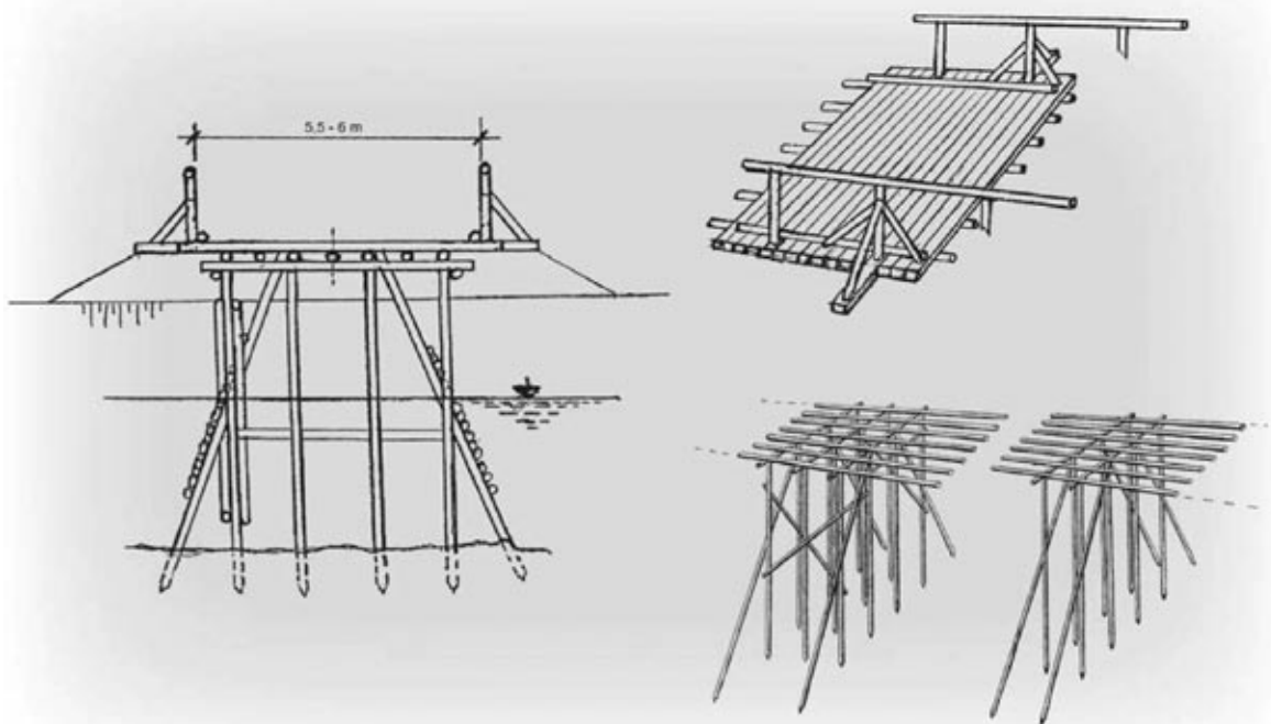
27. kép: Rekonstruált cölöpjárom, járósínt és a cölöpjármok térbeli elhelyezkedése. Fig. 27: Reconstruction of the pile bents, the walkway and a 3D view of the pile bents.
